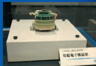
「はやぶさ」再突入カプセル 搭載電子機器部
